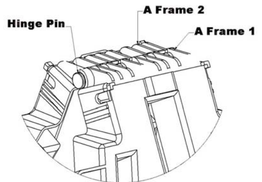
A-Frame Hinge Assembly
